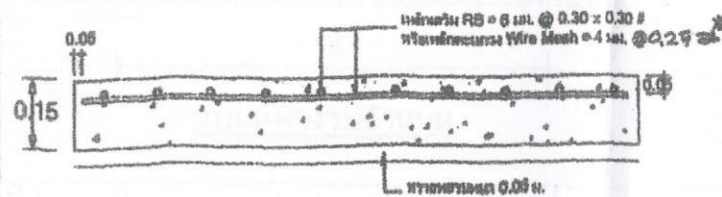
แบบขยายรูปตัดแสดงการเสริมเหล็ก
