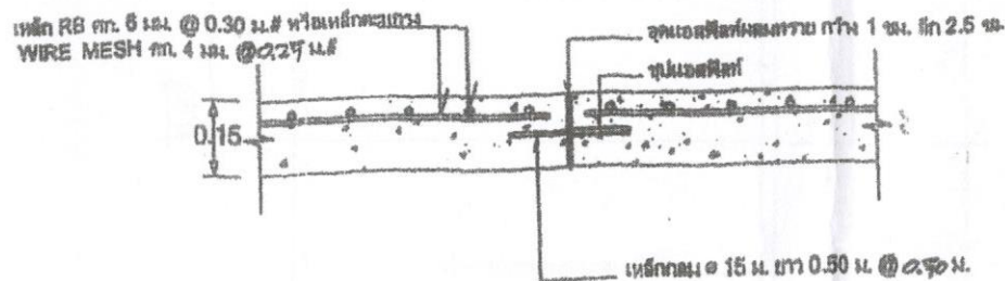
แบบขยาย EXPANSION JOINT (ใช้ความยาว 50.00 ม.)
