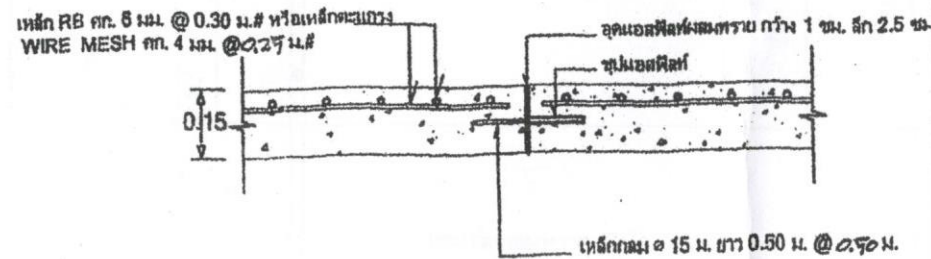
แบบขยาย EXPANSION JOINT (โดยความยาว 50.00 ม.)
