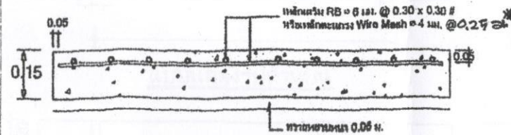
แบบขยายรูปตัดแสดงการเสริมเหล็ก
