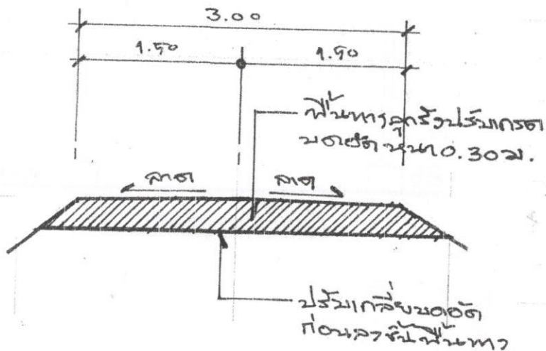
รูปตัดขวางสร้างทาง 1:๕๐
